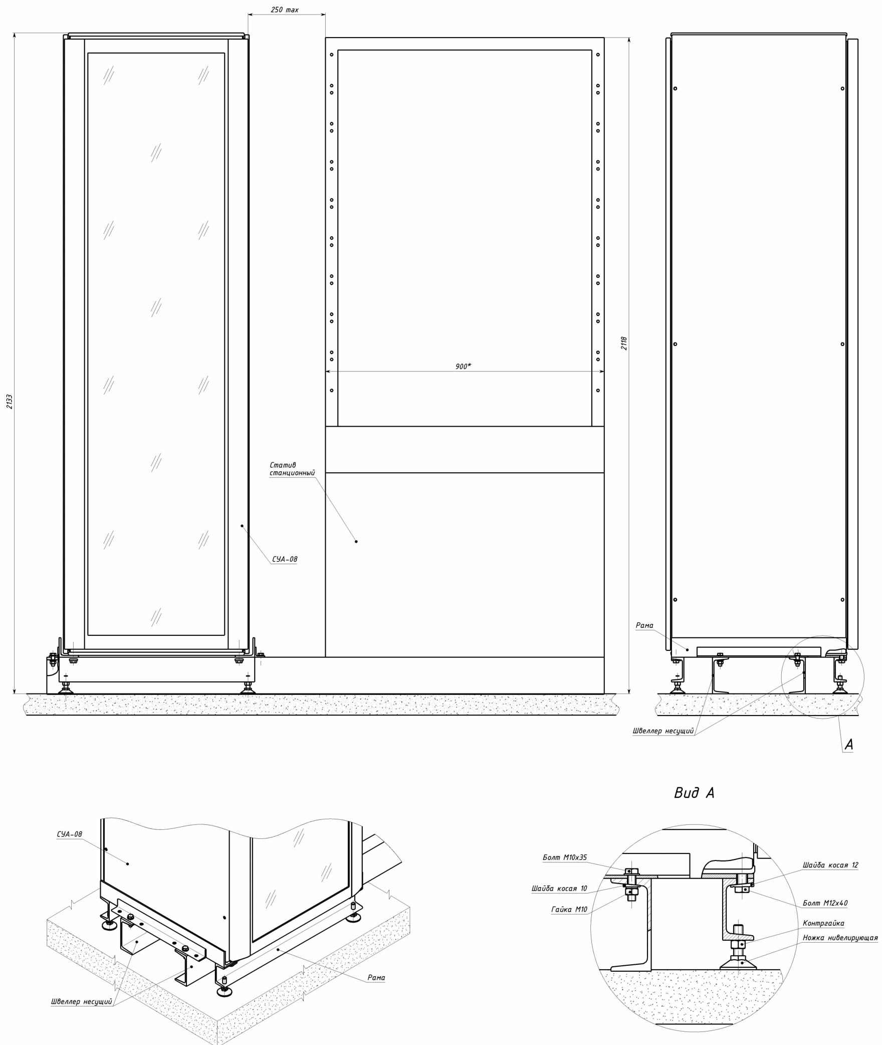
Рис.3. СУА-08. Установка в помещении.
